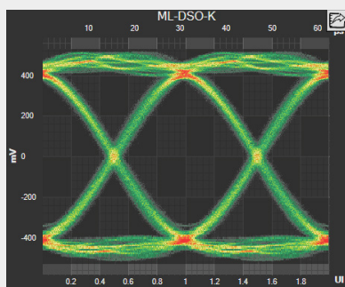
32G NRZ PCIe Gen 5
